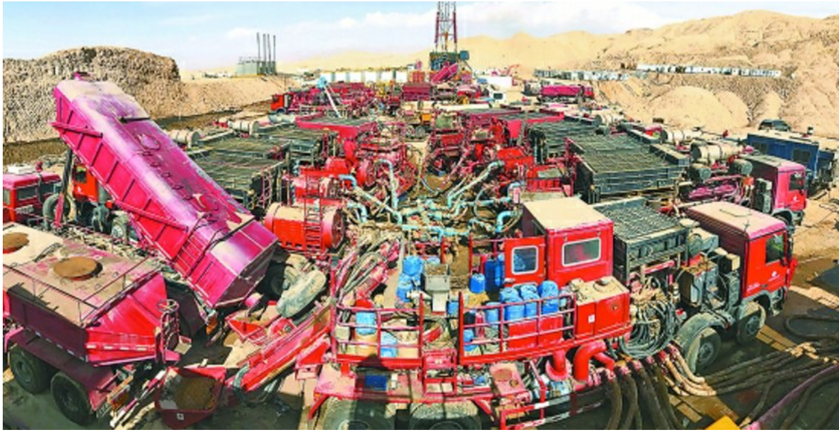
近日,青海油田井下作业公司施工的狮49H1井裸眼分隔器压裂施工圆满收官。
